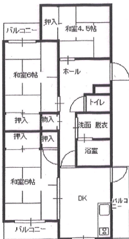
泉が丘1号棟3DKA1右
